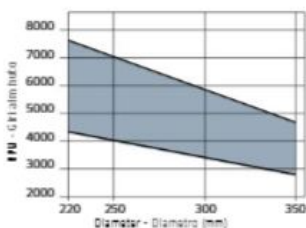
Minimum and maximum RPM based on the blade diameter. Fascia dei R. giri minimo e massimo consigliati in funzione del diametro della lama.
