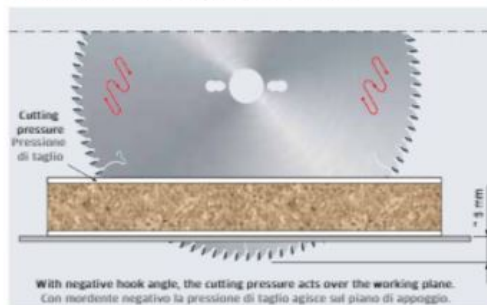
Working with spindle over the working plane Lavorazione con albero sopra il piano di lavoro
