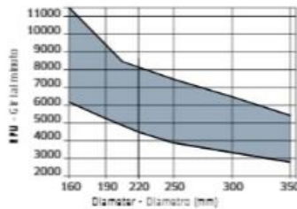
Minimum and maximum RPM based on the blade diameter. Fascia dei N. giri minimo a massimo consigliati in funzione del diametro della lama.
