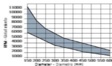
Minimum and maximum RPM based on the blade diameter. Rapporto dei N. giri minimo e massimo consigliati in funzione del diametro della lama.
