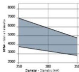
Minimum and maximum RPM based on the blade diameter. Scala dei N. giri minimo e massimo consigliati in funzione del diametro della lama.
