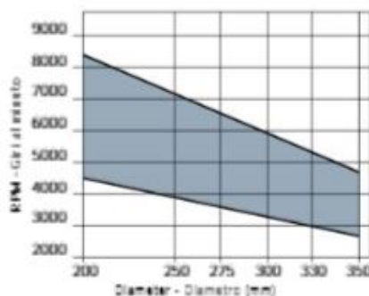
Minimum and maximum RPM based on the blade diameter. Fascia dei R. giri minimo e massimo consigliati in funzione del diametro della lama.
