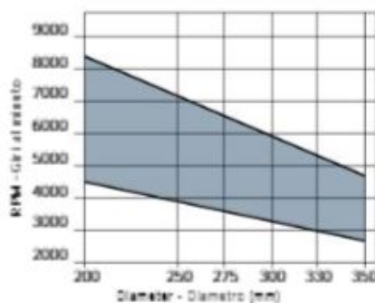
Minimum and maximum RPM based on the blade diameter. Fascia dei N. giri minimo e massimo consigliati in funzione del diametro della lama.
