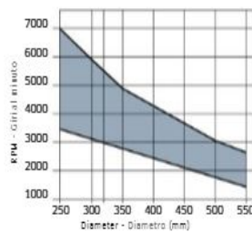
Minimum and maximum RPM based on the blade diameter. Pascia dei giri minimo e massimo consigliati in funzione del diametro della lama.
