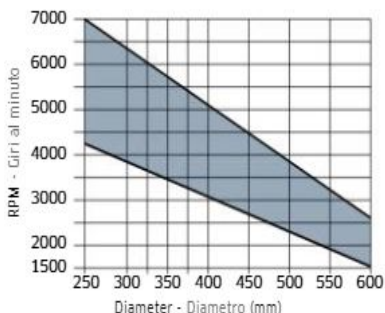
Minimum and maximum RPM based on the blade diameter. Fascia del N. giri minimo e massimo consigliati in funzione del diametro della lama.
