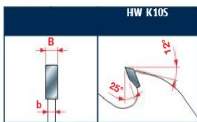
Tooth features - Caratteristiche del dente
