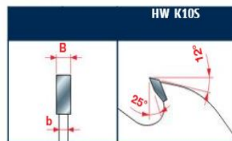
Tooth features - Caratteristiche del dente
