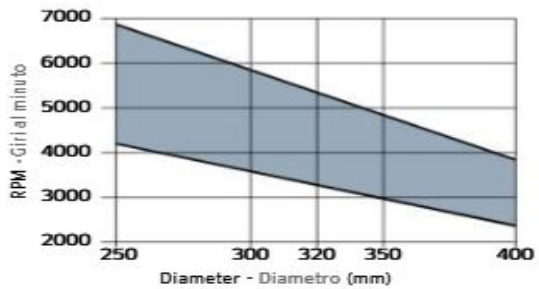
Minimum and maximum RPM based on the blade diameter. Fascia del N. giri minimo e massimo consigliati in funzione del diametro della lama.
