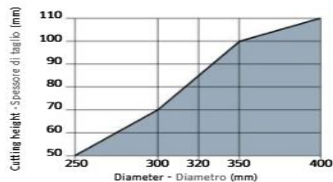
Maximum depth of cut based on the blade diameter. Altezza di taglio massima consentita in funzione del diametro della lama.
