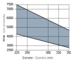
Minimum and maximum RPM based on the blade diameter. Fascia del N. giri minimo e massimo consigliati in funzione del diametro della lama.
