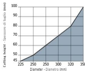
Maximum depth of cut based on the blade diameter. Altezza di taglio massima consentita in funzione del diametro della lama.
