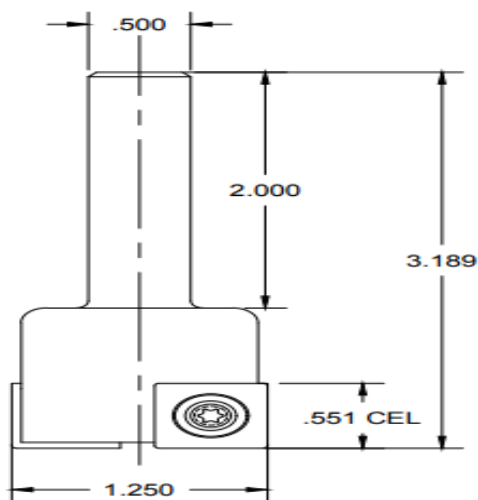
8300 INSERT TOOL
